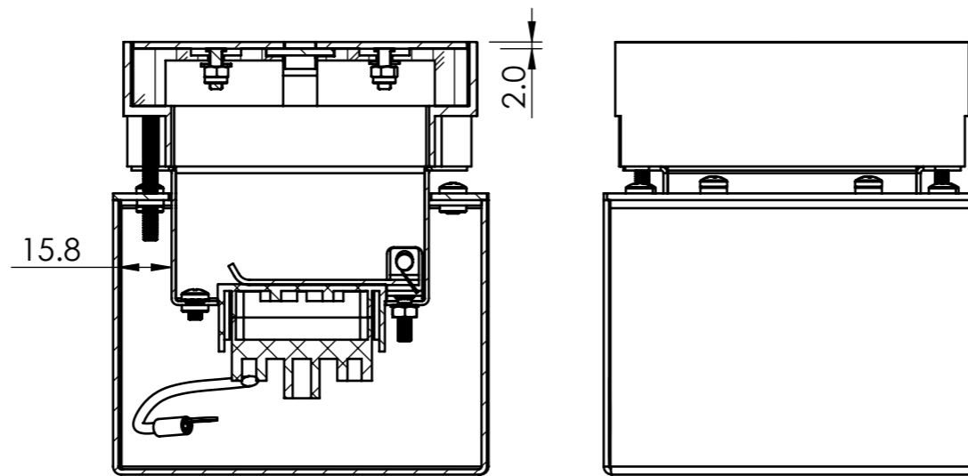
SECTION A-A
