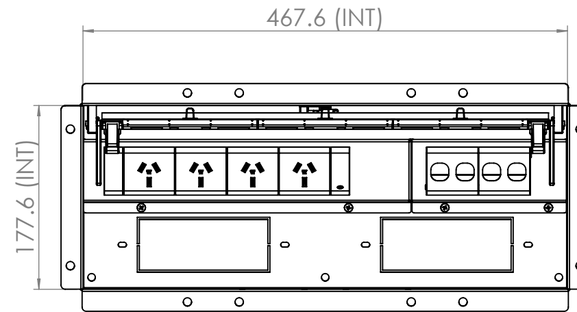
TOP VIEW - LID OPEN
